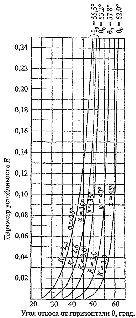
Рисунок В.4 – Графики для определения крутизны откоса при 2 < K \leq 3
