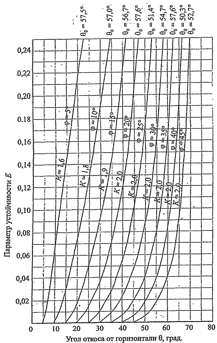
Рисунок В.3 — Графики для определения крутизны откоса при 1 < K \leq 2
